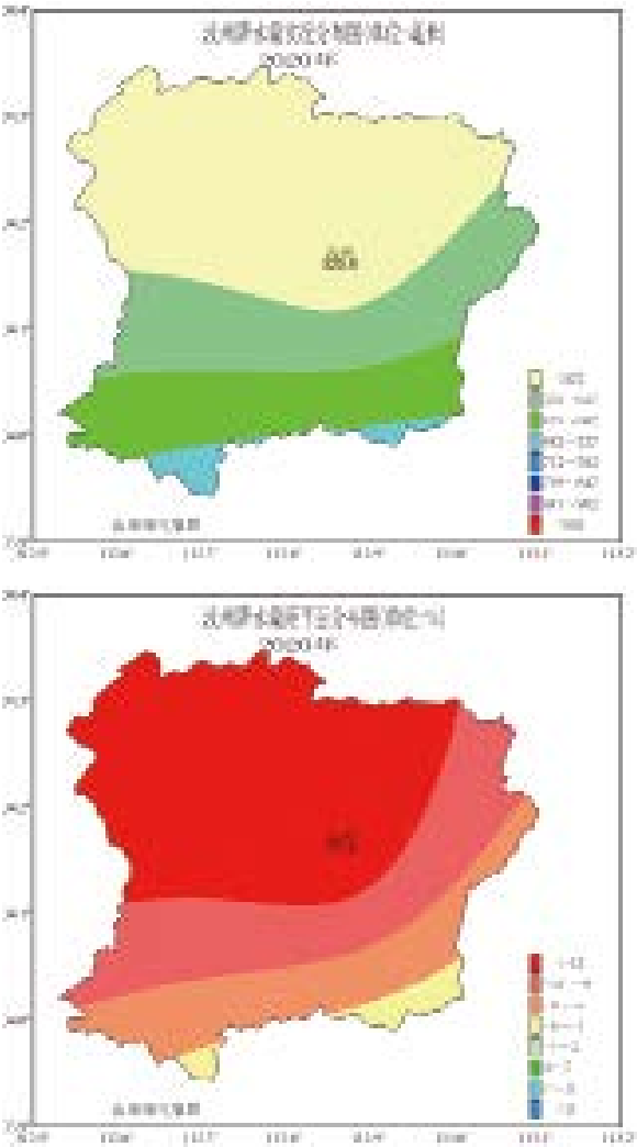
图 4:2020 年降水（20—20）（左）及距平百分率（右）分布图
